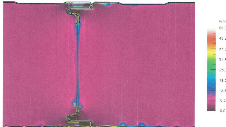
Wärmestromdichte an der Stoßfuge am Beispiel Wand ISOPAR ®
